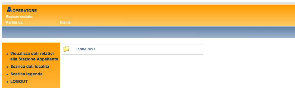
Figura 1.3: Pagina principale
