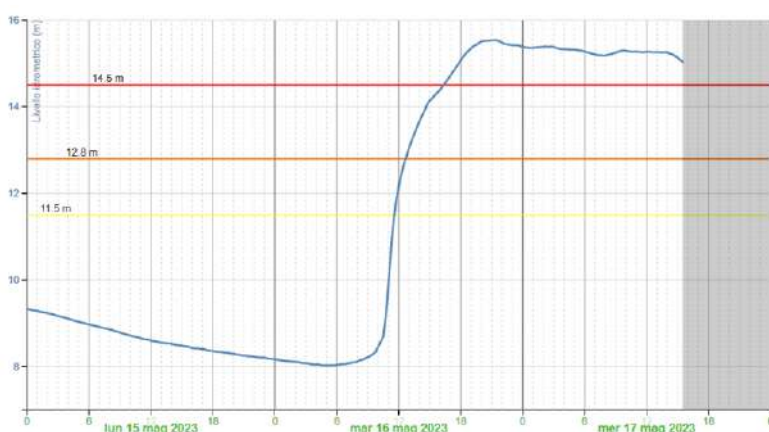
Figura 5 - Idrogramma di piena registrato alla stazione idrometrica di Sesto Imolese sul Sillaro. FONTE ARPAE Emilia Romagna
